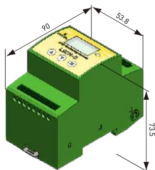
Caja de monitoreo LSCM-D/24
