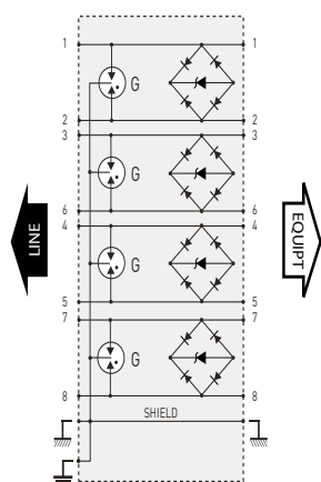
G : Descargador de gas tripolar
