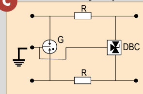
C Protección baja capacidad
