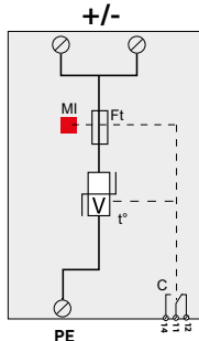
DS250E-48DC
