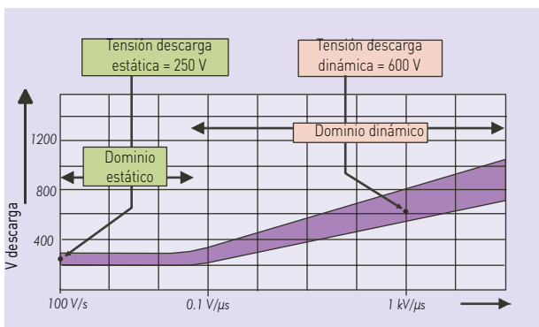
Tensiones de descarga estáticas y dinámicas
