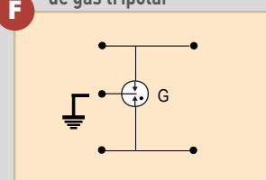
F Protección con descargador de gas tripolar
