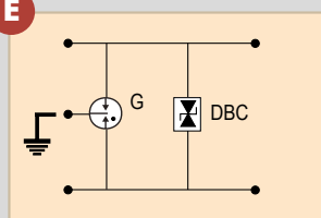
E Protección alta velocidad
