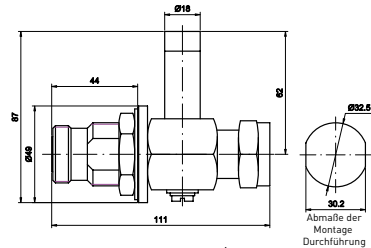
PRC822S-716W/MF
