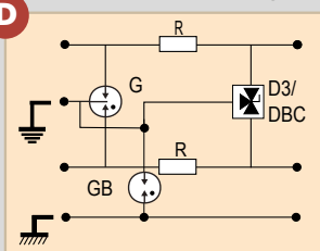
D Protección con blindaje
