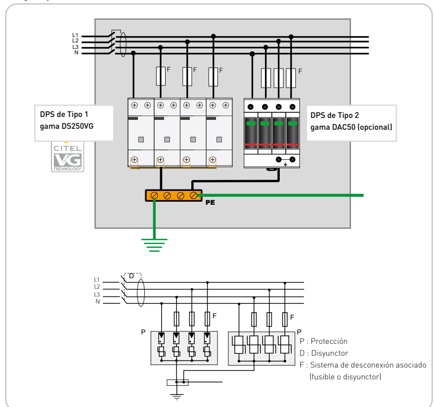
Ejemplo de coordinación en una red trifásica
