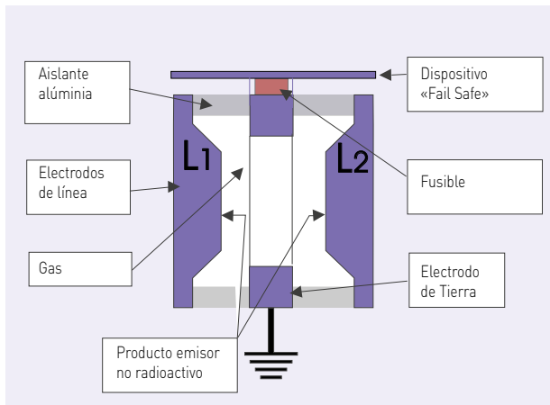
Descargador Tripolar
