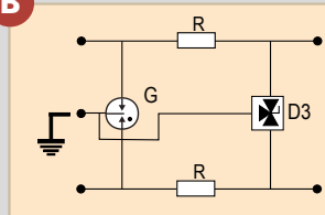
B Protección reforzada
