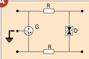
A Protección estándar
